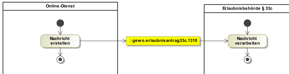
Abbildung III.4.2. Ablauf Übermittlung eines Antrags auf Bestätigung des Aufstellorts gemäß § 33c Absatz 3 GewO
