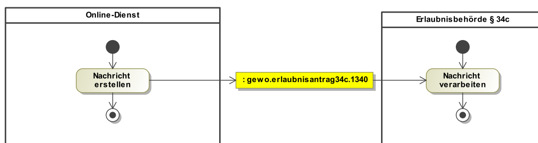
Abbildung III.7.1. Ablauf Übermittlung eines Erlaubnisantrags nach § 34c GewO
