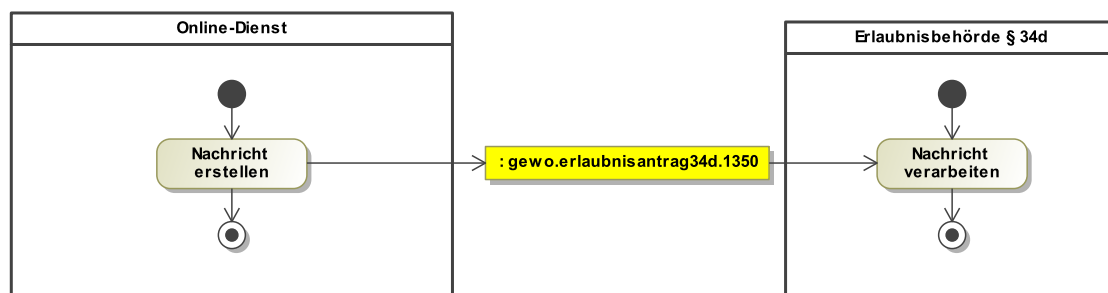
Abbildung III.8.1. Ablauf Übermittlung eines Erlaubnisantrags nach § 34d GewO
