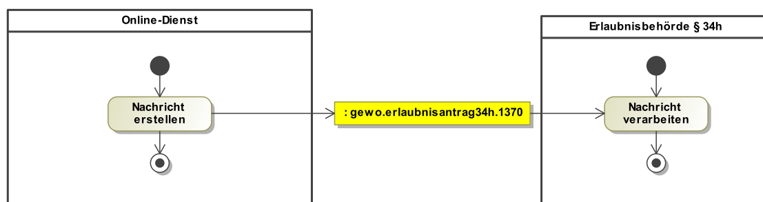
Abbildung III.10.1. Ablauf Übermittlung eines Erlaubnisantrags nach § 34h GewO
