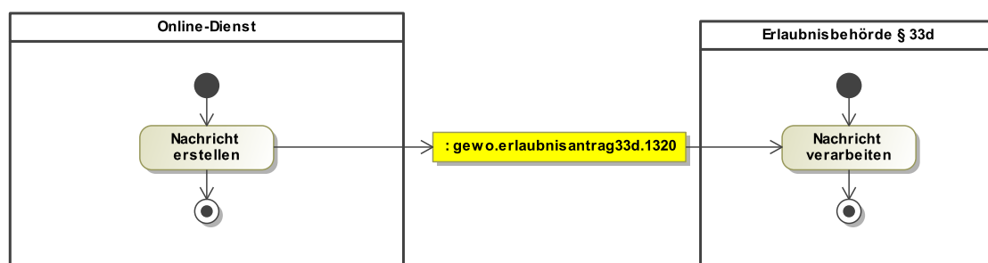
Abbildung III.5.1. Ablauf Übermittlung eines Erlaubnisantrags nach § 33d GewO
