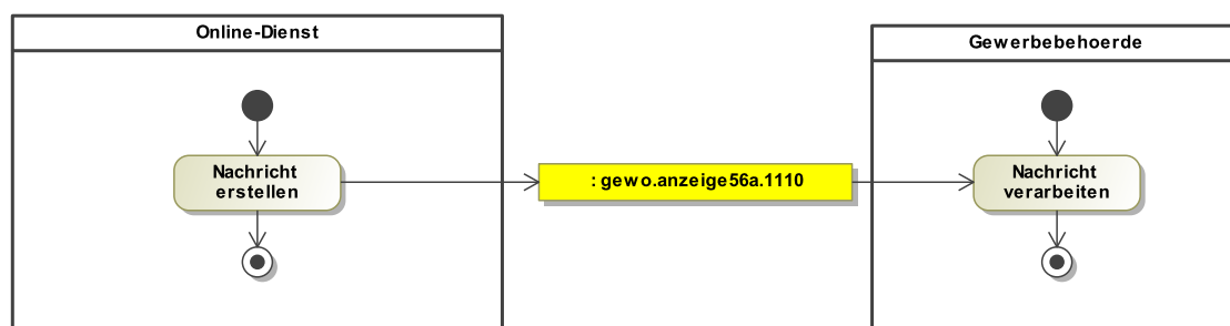
Abbildung III.3.1. Ablauf Übermittlung einer Anzeige nach § 56a GewO
