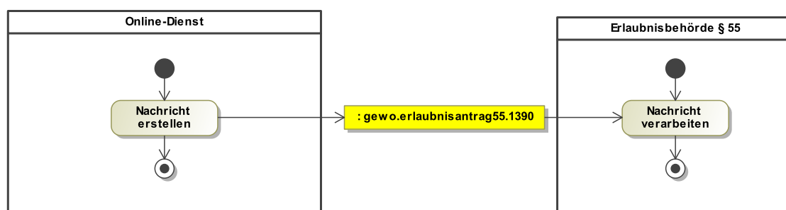
Abbildung III.12.1. Ablauf Übermittlung eines Erlaubnisantrags nach § 55 GewO
