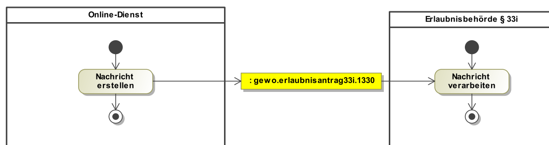
Abbildung III.6.1. Ablauf Übermittlung eines Erlaubnisantrags nach § 33i GewO
