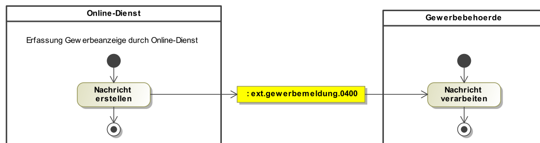
Abbildung II.18.2. Ablauf Übermittlung einer Gewerbeanzeige durch einen Online-Dienst an die zuständige Gewerbebehörde
