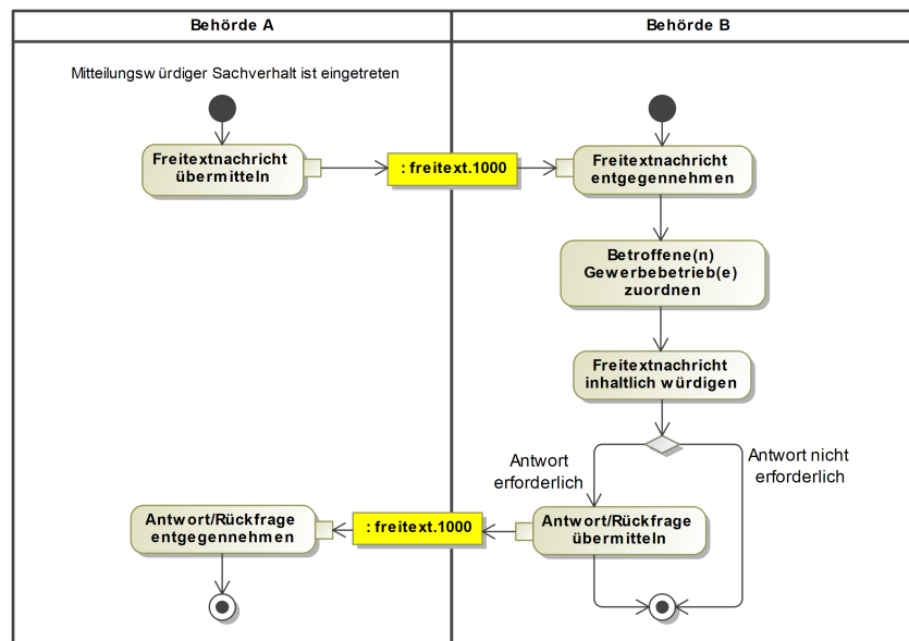
Abbildung I.7.2. Ablauf zur Übermittlung einer Freitextnachricht
