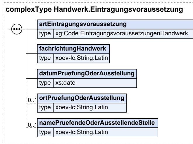
Abbildung V.3.2. Handwerk.Eintragungsvoraussetzung
