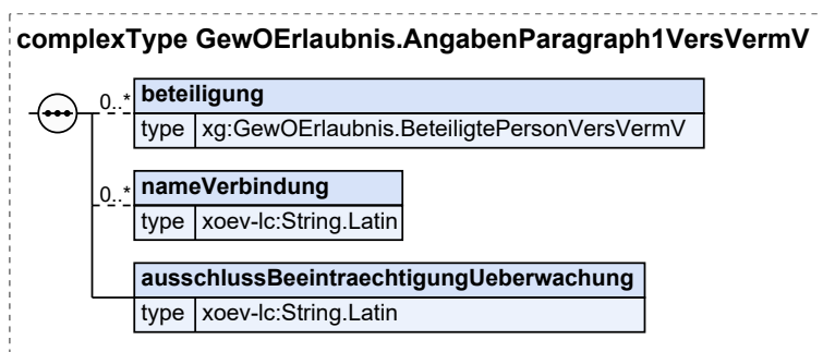
Abbildung IV.3.1. GewOErlaubnis.AngabenParagraph1VersVermV
