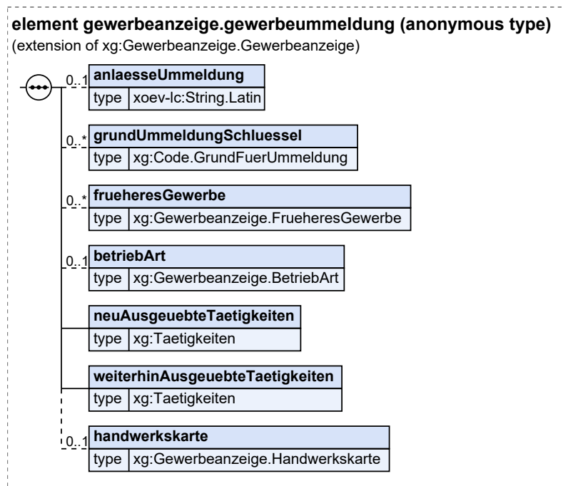
Abbildung III.2.2. gewerbeanzeige.gewerbeummeldung
