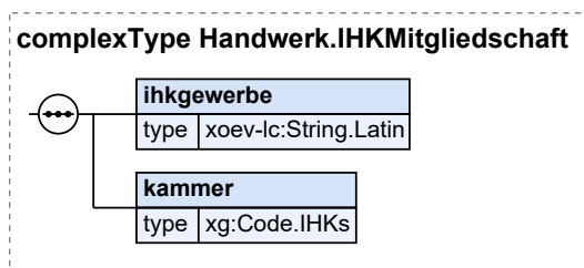
Abbildung V.3.3. Handwerk.IHKMitgliedschaft
