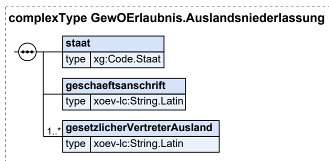
Abbildung IV.3.3. GewOErlaubnis.Auslandsniederlassung
