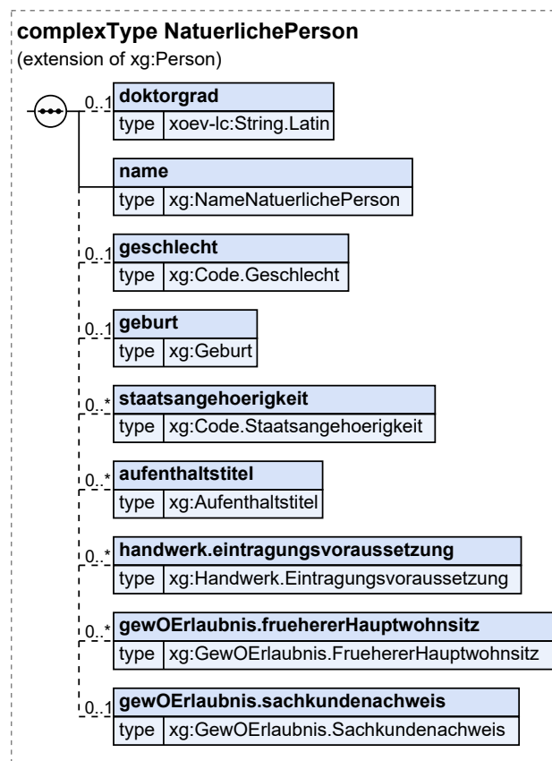
Abbildung II.4.3. NatuerlichePerson
