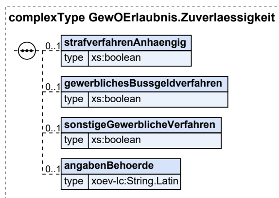
Abbildung IV.3.10. GewOErlaubnis.Zuverlaessigkeit
