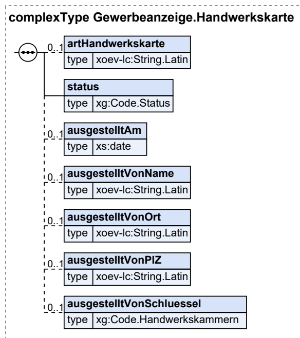
Abbildung III.3.5. Gewerbeanzeige.Handwerkskarte
