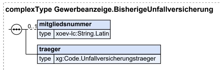
Abbildung III.3.2. Gewerbeanzeige.BisherigeUnfallversicherung
