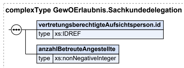
Abbildung IV.3.7. GewOErlaubnis.Sachkundedelegation
