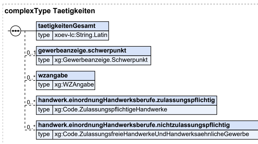
Abbildung II.5.1. Taetigkeiten
