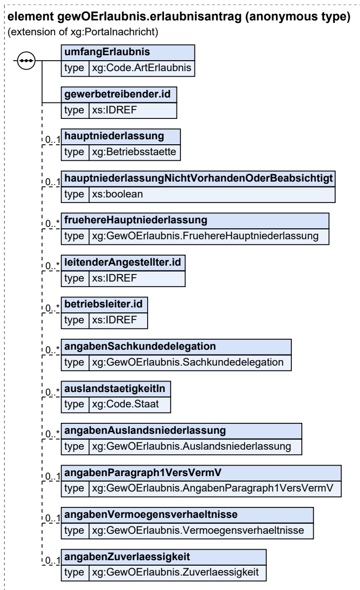
Abbildung IV.2.1. gewOErlaubnis.erlaubnisantrag
