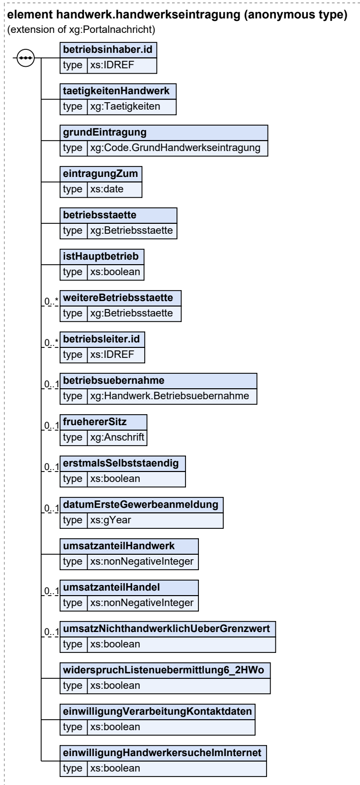
Abbildung V.2.1. handwerk.handwerkseintragung
