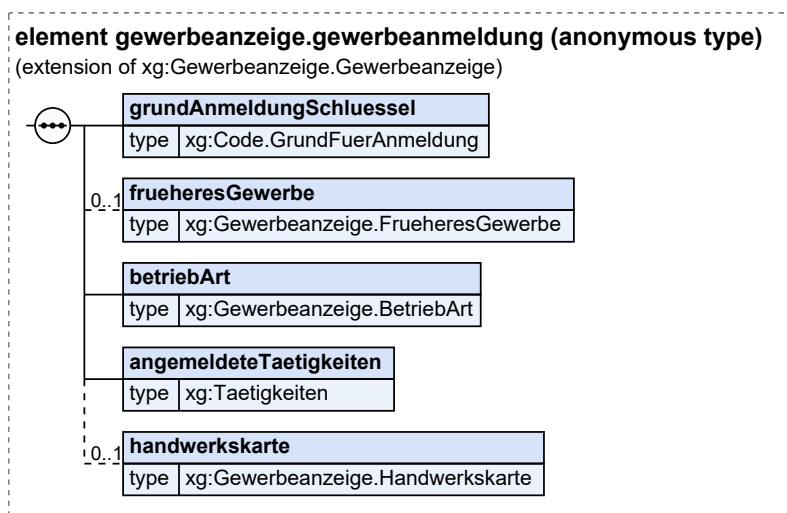
Abbildung III.2.1. gewerbeanzeige.gewerbeanmeldung
