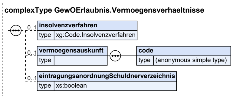
Abbildung IV.3.9. GewOErlaubnis.Vermögensverhältnisse
