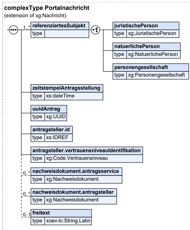
Abbildung II.3.7. Portalnachricht
