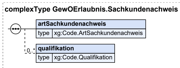
Abbildung IV.3.8. GewOErlaubnis.Sachkundenachweis
