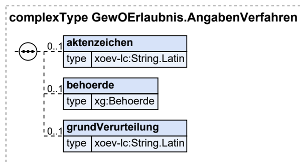
Abbildung IV.3.2. GewOErlaubnis.AngabenVerfahren
