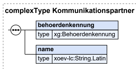
Abbildung II.3.4. Kommunikationspartner
