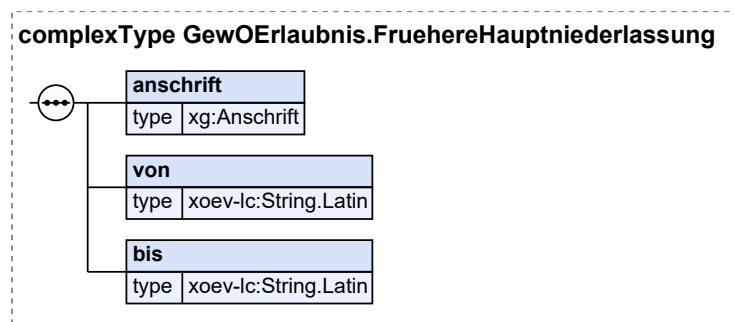
Abbildung IV.3.6. GewOErlaubnis.FruehereHauptniederlassung
