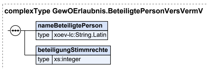
Abbildung IV.3.4. GewOErlaubnis.BeteiligtePersonVersVermV
