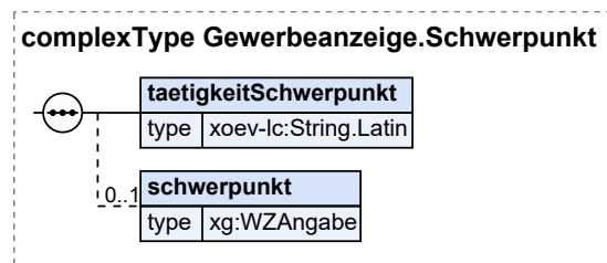
Abbildung III.3.7. Gewerbeanzeige.Schwerpunkt
