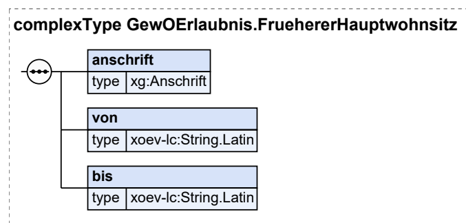
Abbildung IV.3.5. GewOErlaubnis.FruehererHauptwohnsitz
