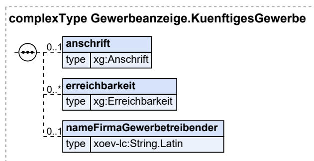
Abbildung III.3.6. Gewerbeanzeige.KuenftigesGewerbe
