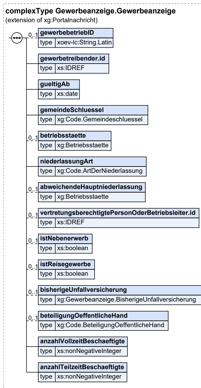
Abbildung III.3.4. Gewerbeanzeige.Gewerbeanzeige
