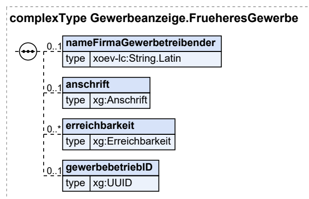
Abbildung III.3.3. Gewerbeanzeige.FrueheresGewerbe
