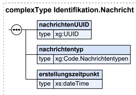
Abbildung II.3.2. Identifikation.Nachricht
