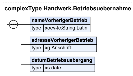
Abbildung V.3.1. Handwerk.Betriebsuebernahme
