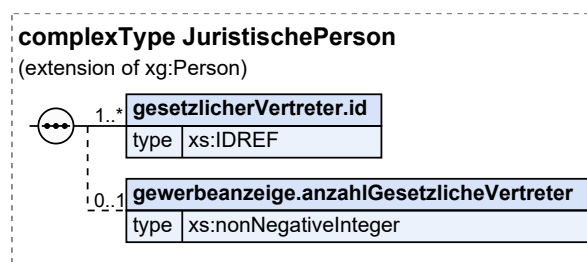
Abbildung II.4.2. JuristischePerson
