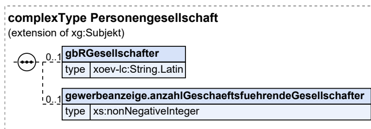
Abbildung II.4.5. Personengesellschaft
