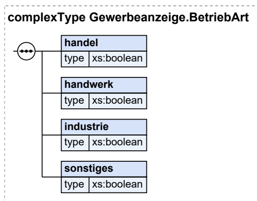
Abbildung III.3.1. Gewerbeanzeige.BetriebArt
